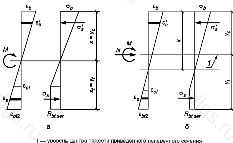
Рисунок 8.17 — Схема напряженно-деформированного состояния сечения элемента при проверке образования трещин при действии изгибающего момента (а), изгибающего момента и продольной силы (б)
