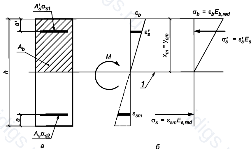
Рисунок 8.19 — Приведенное поперечное сечение (а) и схема напряженно-деформированного состояния элемента с трещинами (б) для расчета его по деформациям при действии изгибающего момента
