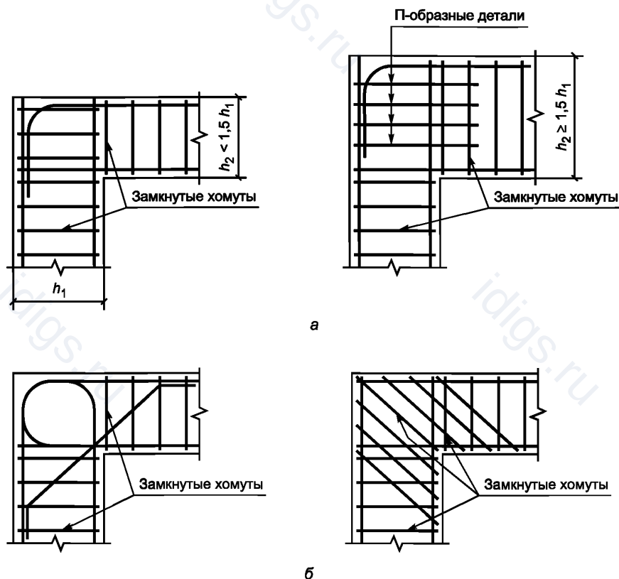
Рисунок 10.2 — Узлы сопряжения балок с колоннами
