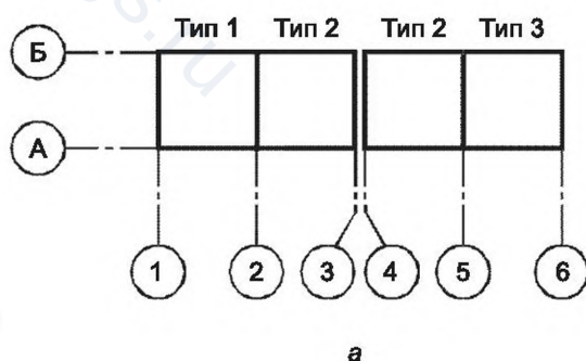
Рисунок 4 — Примеры присвоения обозначений и размещения координационных осей блок-секций
