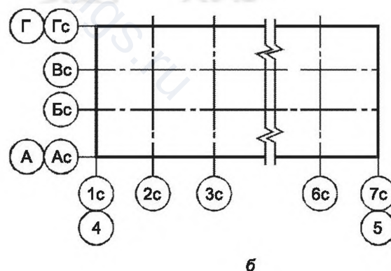
Рисунок 4 — Примеры присвоения обозначений и размещения координационных осей блок-секций
